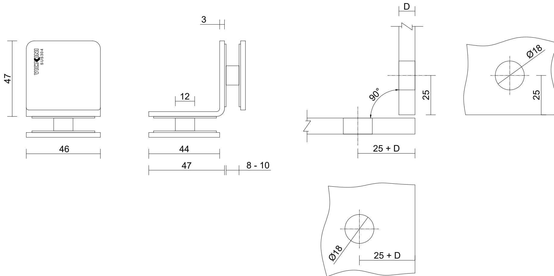
Thông số khoan lỗ trên kính
